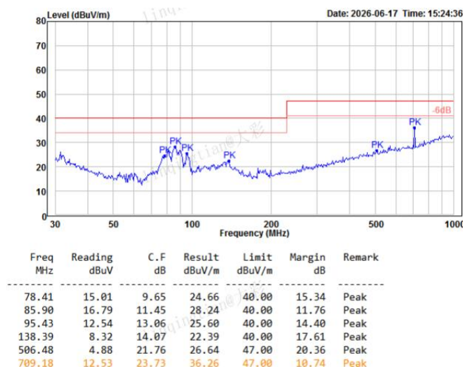
图 4-7 RE 测试垂直方向
