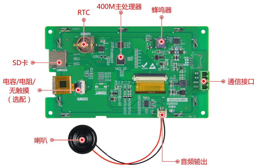
图 1-4 硬件配置图
