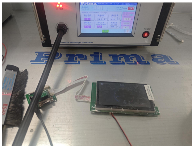
图 4-2 ESD 测试图
