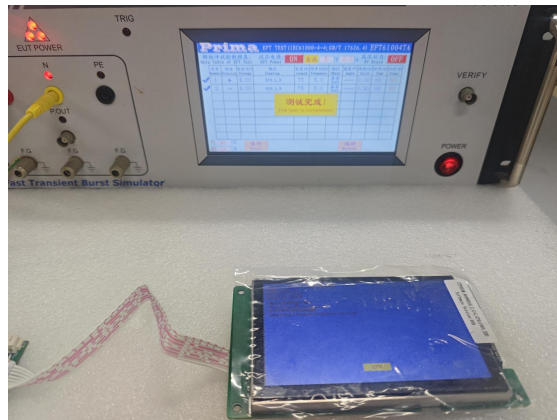
图 4-3 EFT 测试图
