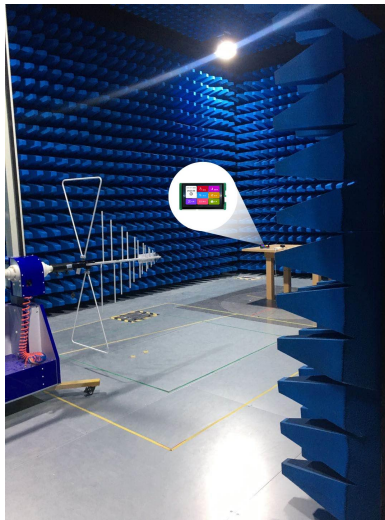
图 4-5 RE 测试图
