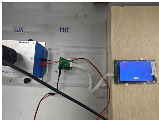
图 4-4 CS 测试图
