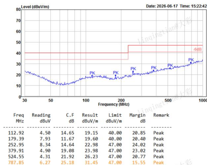
图 4-6 RE 测试水平方向
